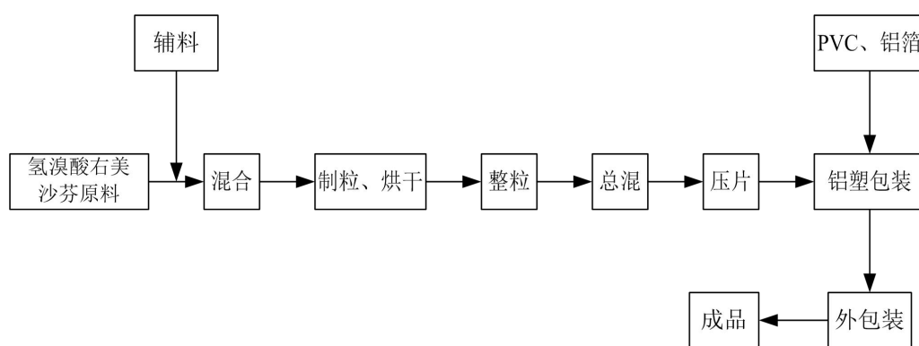
图4-1 制剂车间片剂生产工艺
